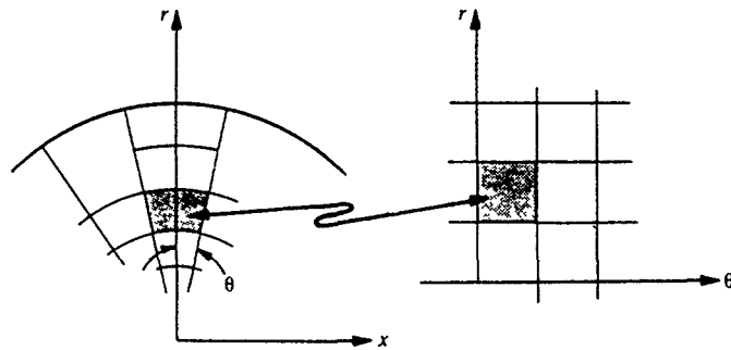
Figura 11.3 Transformación polar de coordenadas.
