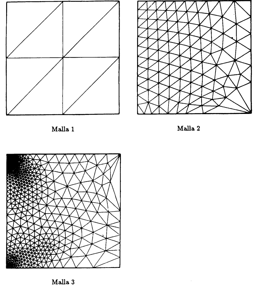
Figura 14.6 Malla adaptable de elementos triangulares lineales para la viga corta en voladizo.
