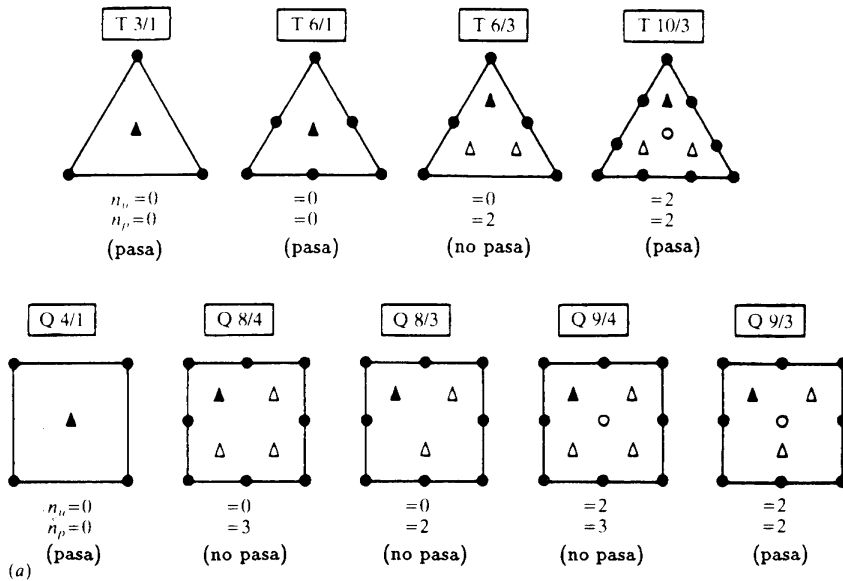
Figura 12.7(a) Formulación u – p para elasticidad incompresible. Aproximación discontinua de la presión. (a) Tests de la parcela para un solo elemento. (b) Tests de la parcela para varios elementos.
