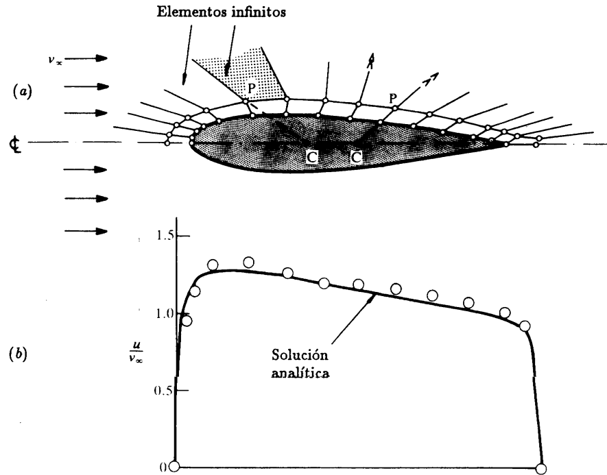
Figura 8.21 Flujo irrotacional alrededor de la sección de ala NACA0018. 29 (a) Malla de elementos isoparamétricos bilineales y elementos infinitos. (b) Resultados para la velocidad paralela a la superficie. Calculados y —analíticos.
