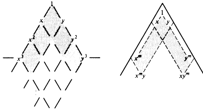
Figura 7.12 Términos generados por funciones de forma de borde en los elementos serendípticos ( 3 \times 3 y m \times m ).
