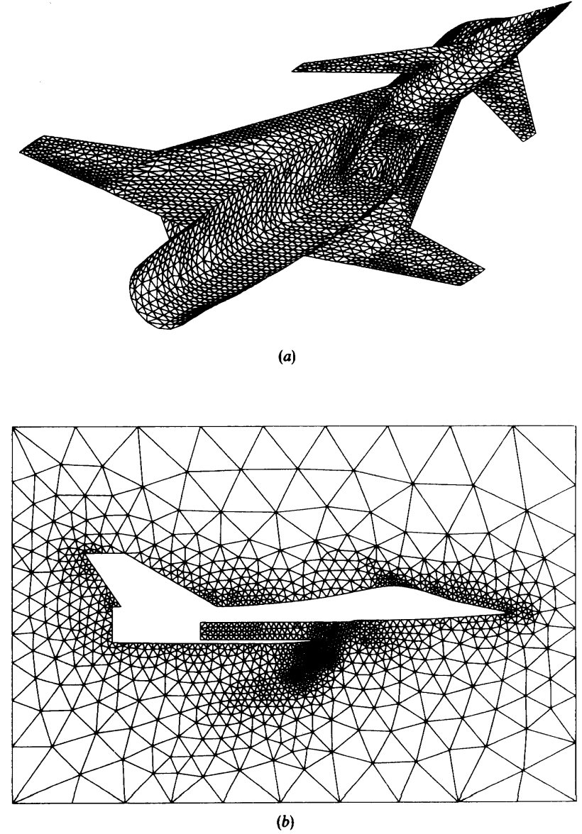
Figura 5.8 (a) Malla de tetraedros en la región exterior generada automáticamente especificando la densidad de mado y (b) intersección de la malla con el plano central del avión.
