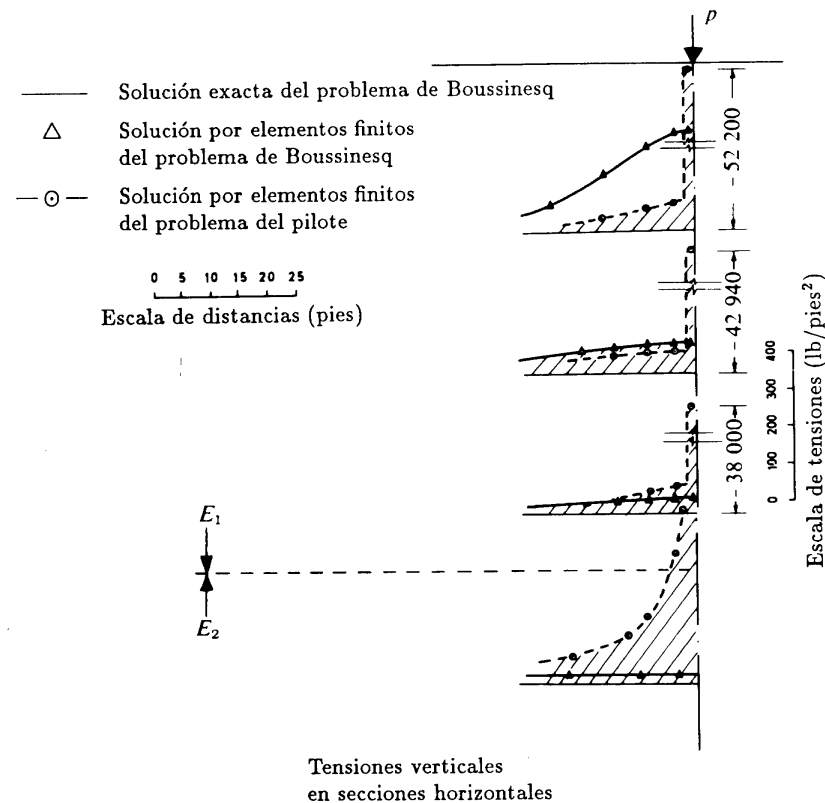
Figura 4.9 (b) Pilote en terreno estratificado. Gráfico de las tensiones verticales en secciones horizontales. Gráfico también de la solución para el problema de Boussinesq obtenida haciendo E_1 = E_2 = E_{\text{pilote}} y comparación de ésta con los valores exactos.
