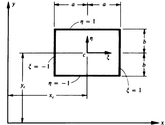
Figura 7.4 Coordenadas normalizadas para un rectángulo.
