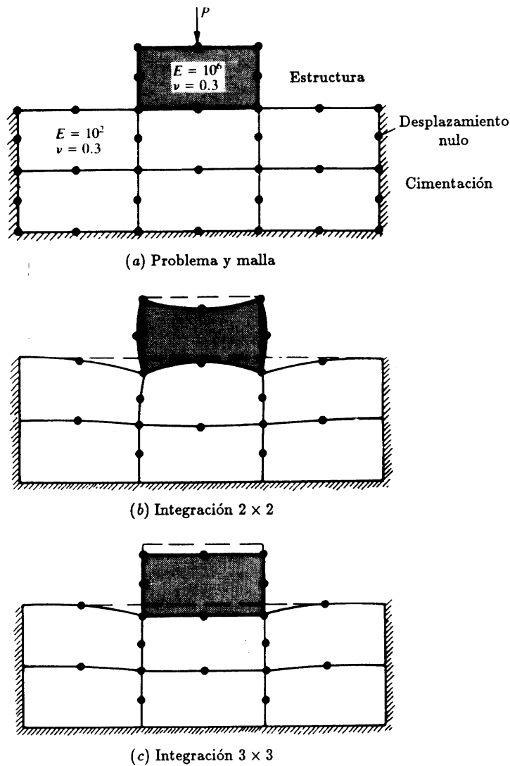
Figura 11.8 Propagación de un modo espúreo a partir de un único elemento no satisfactorio.
