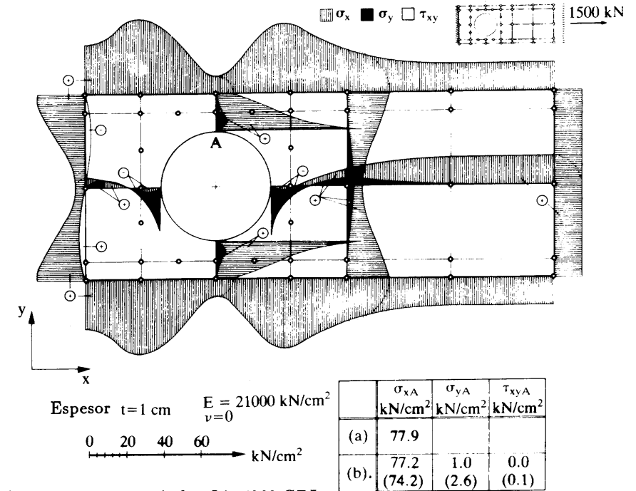
(b) 920 elementos estándar Q8, 5960 GDL
