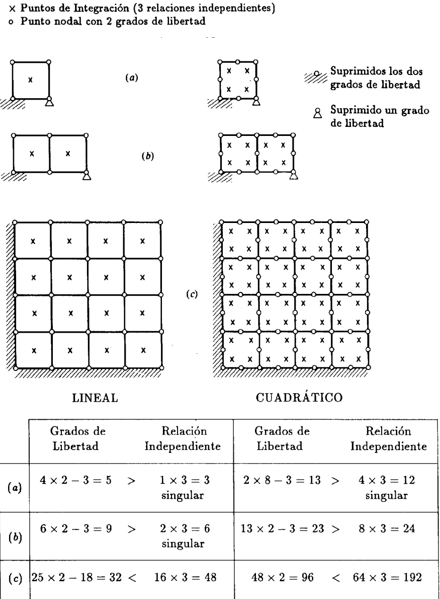
Figura 8.14 Comprobación de la singularidad de la matriz en problemas de elasticidad bidimensional (a), (b) y (c).
