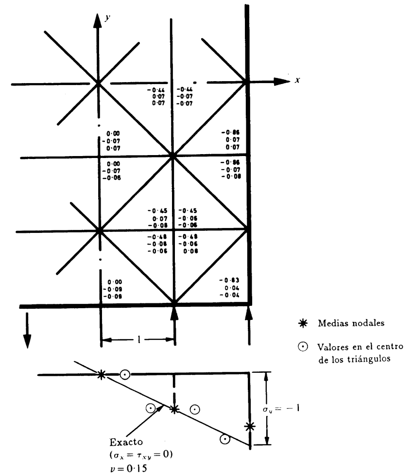
Figura 3.4 Flexión pura de una viga resuelta mediante una malla no tupida de elementos triangulares (se reseñan los valores de \sigma_y , \sigma_x y \tau_{xy} por este orden).
