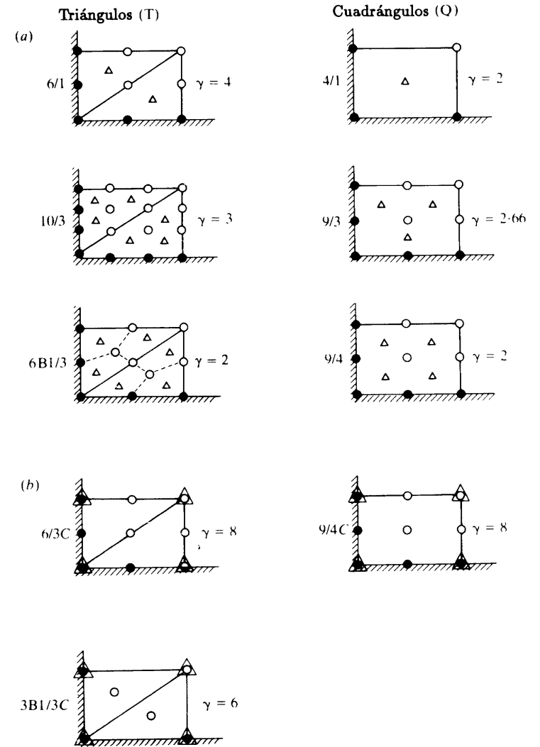
Figura 12.11 El índice de libertad o relación de parcela infinita para varios elementos u - p para elasticidad incompresible ( \gamma = n_u/n_p ). (a) Presión discontinua. (b) Presión continua.
