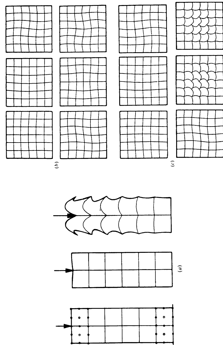
Figura 11.9 Respuesta peculiar de ensamblajes de elementos casi singulares 17 . (a) Una columna de elementos de nueve nodos con carga puntual para integraciones 3 x 3 y 2 x 2. El ensamblaje completo es no singular, pero son evidentes modos singulares elementales. (b) Un ensamblaje totalmente coartado de elementos de nueve nodos sin singularidades - los primeros seis modos propios con integración completa (3 x 3). (c) como (b) pero con integración 2 x 2. Nótese la aparición de modos salvajes llamados modos de Esher en la referencia 17 en honor a dicho artista gráfico.
