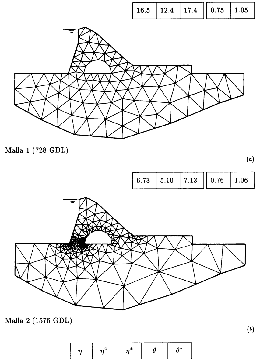
Figura 14.15 Triángulo cuadrático. Generación automática de malla para alcanzar el 5 por ciento de precisión. Análisis de deformación plana de una presa con una cavidad bajo carga de agua solamente. (a) Malla original. (b) Malla refinada. Con la estrategia de refinamiento de la Ec. (14.32) se alcanza, en una operación, una precisión del 4.88 por
