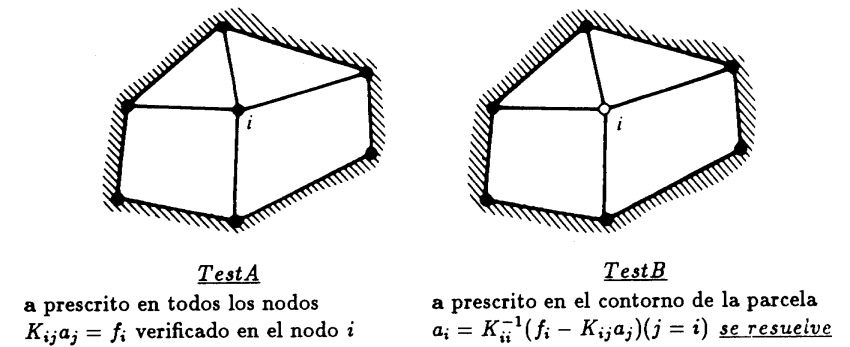
Figura 11.2 Test de la parcela en las formas A y B.
