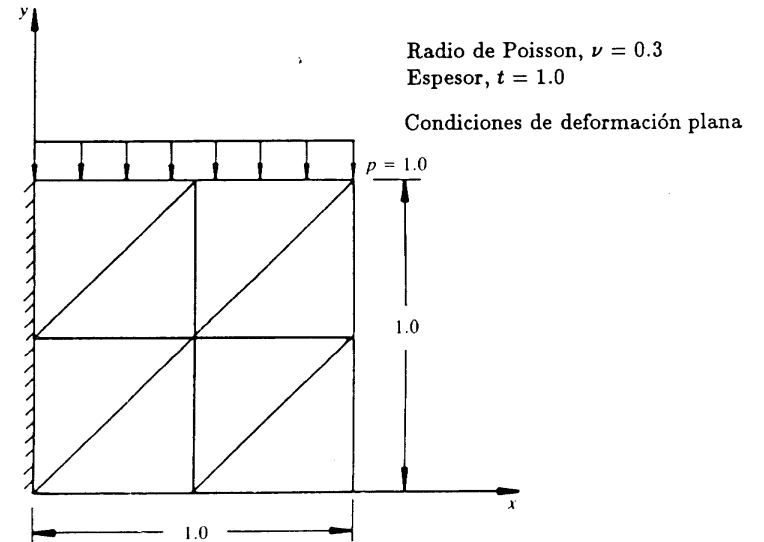
Figura 14.4 Viga corta en voladizo.
