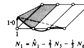
Figura 7.11 Funciones de forma para un elemento "serendípita" de transición cúbico/lineal.
