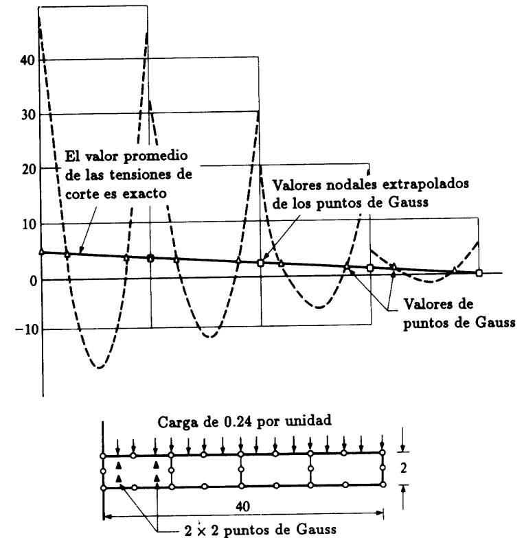
Figura 12.14 Viga en voladizo con cuatro elementos cuadriláteros (Q8). Muestreo de tensiones en los puntos de Gauss de orden cúbico en (2 \times 2) con extrapolación a los nodos.
