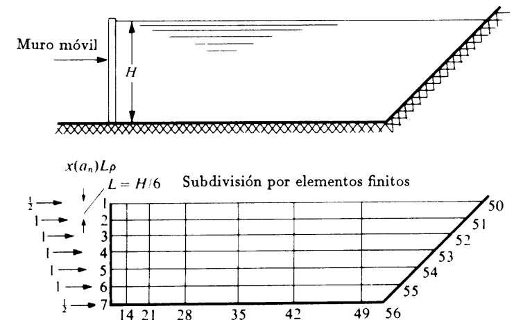
Figura 10.9 Problema de un muro que se desplaza horizontalmente en un depósito.
