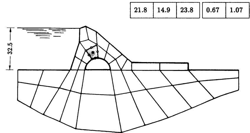
Malla 1 (310 GDL)
