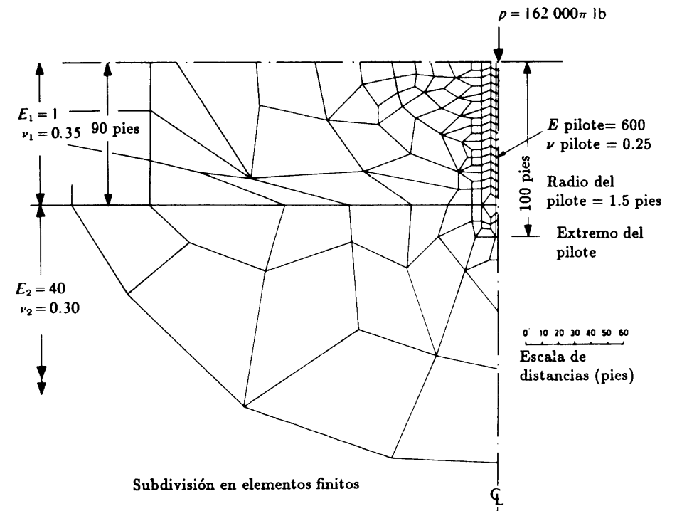
Figura 4.9 (a) Pilote en terreno estratificado. Malla irregular y datos del problema.
