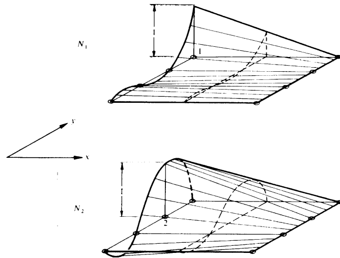
Figura 7.3 Funciones de forma para los elementos de la Figura 7.2.
