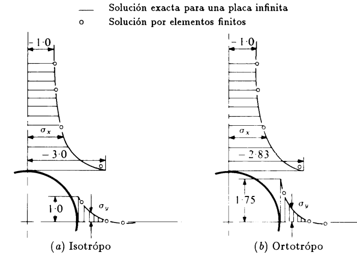
Figura 3.6 Comparación de los resultados teóricos y mediante elementos finitos para los casos (a) y (b) de la Figura 3.5.
