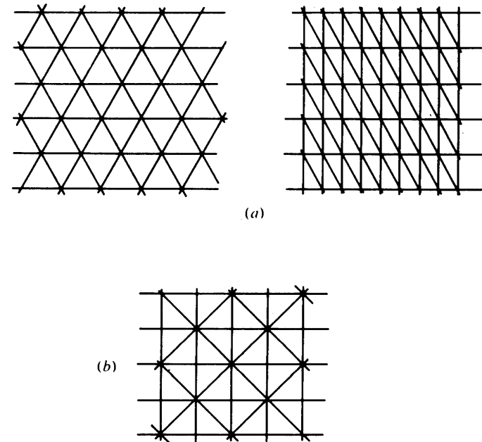
Figura 10.3 Formas de subdivisión “regular” e “irregular”.
