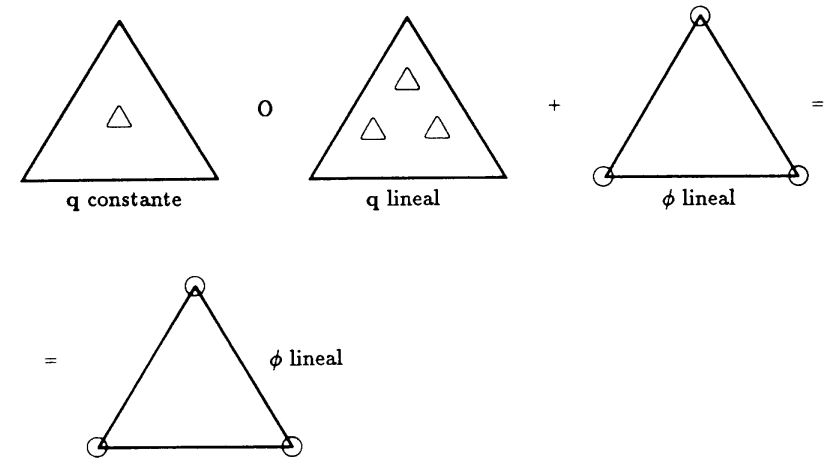
Figura 12.1 Una aproximación mixta al problema de transmisión de calor que produce resultados idénticos que la forma irreducible correspondiente (se supone \mathbf{k} constante en cada elemento).
