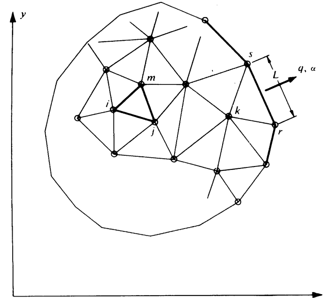
Figura 10.2 División de una región bidimensional en elementos triangulares.
