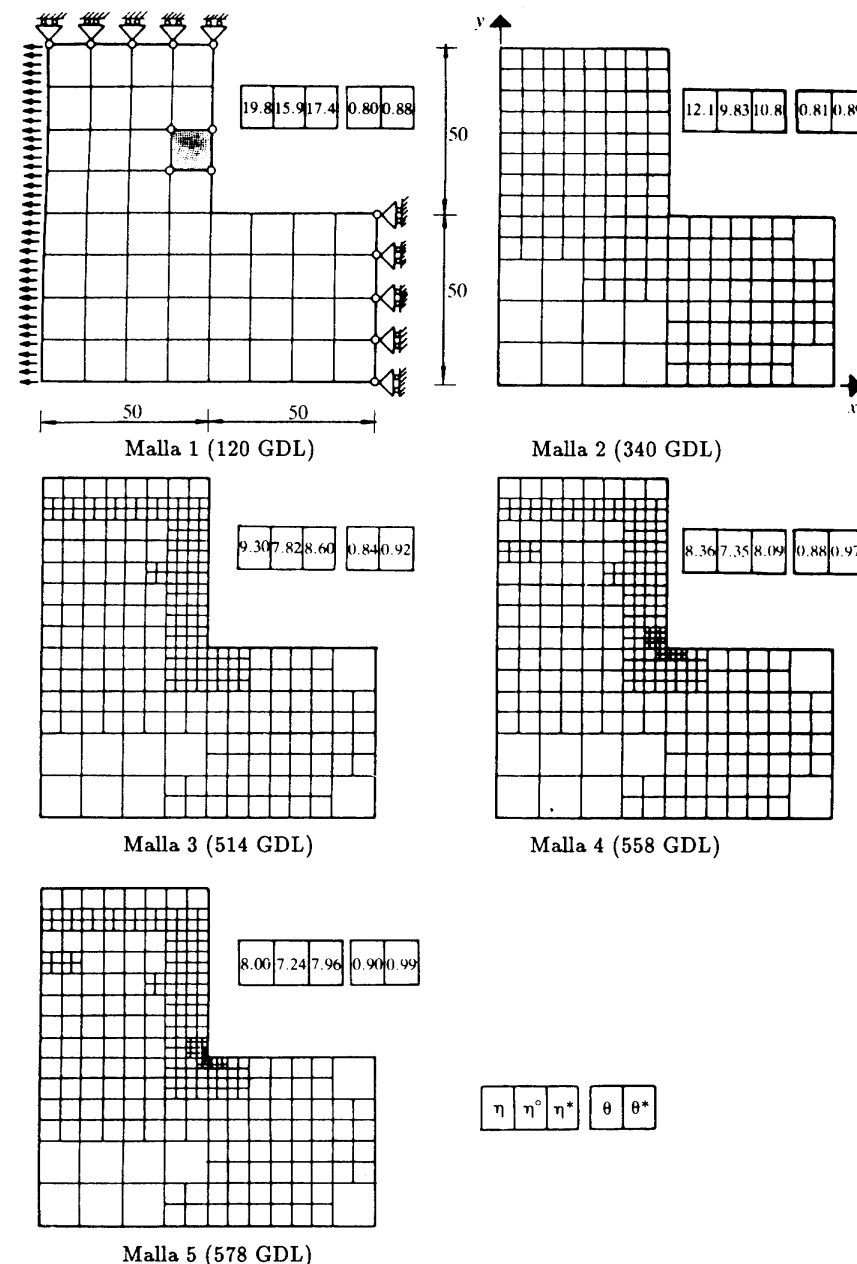
Figura 14.9 Elementos bilineales. Una región en forma de L en tensión plana. Secuencia de refinamiento de malla.
