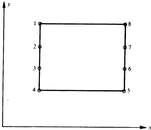
Figura 7.2 Elemento rectangular.
